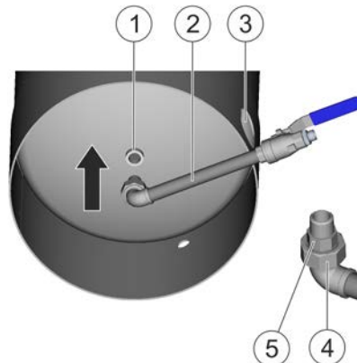
Fig. 19 : Visser la sortie de matière inférieure
