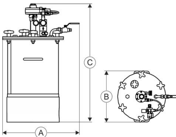
Fig. 60 : Dimensions (variante 2)
