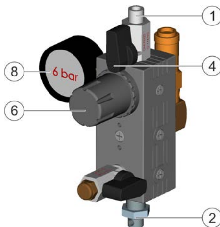
Fig. 9 : Robinetterie d'arrivée d'air comprimé (standard)
